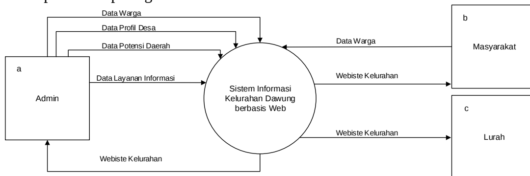
Gambar 2. Desain Context Diagram Sistem Informasi Kelurahan
